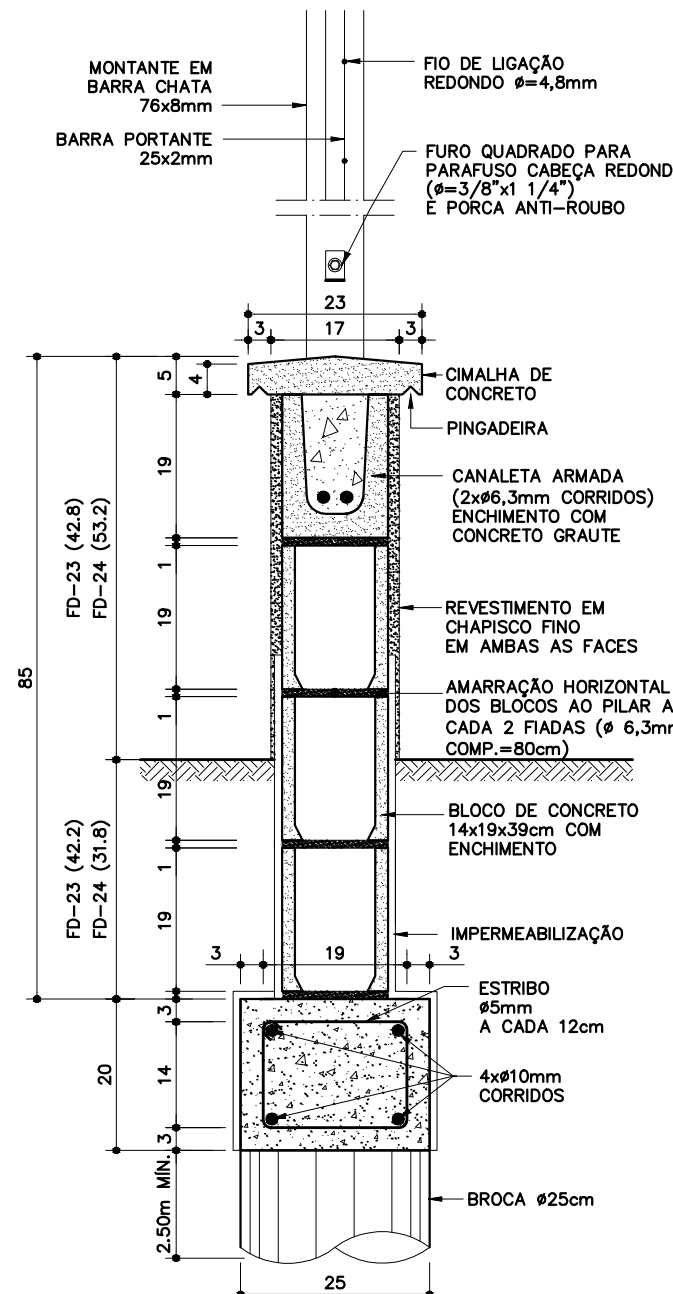
DETALHE 2 ESC. 1:10
