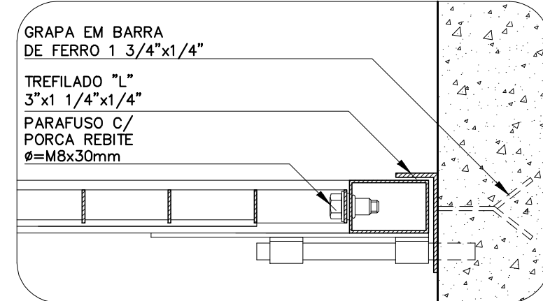
DETALHE 1 PT-33
