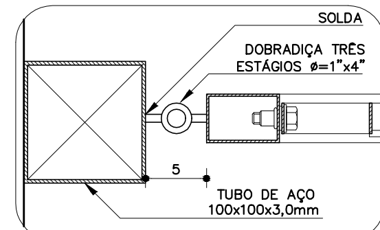
DETALHE 1 PT-35
