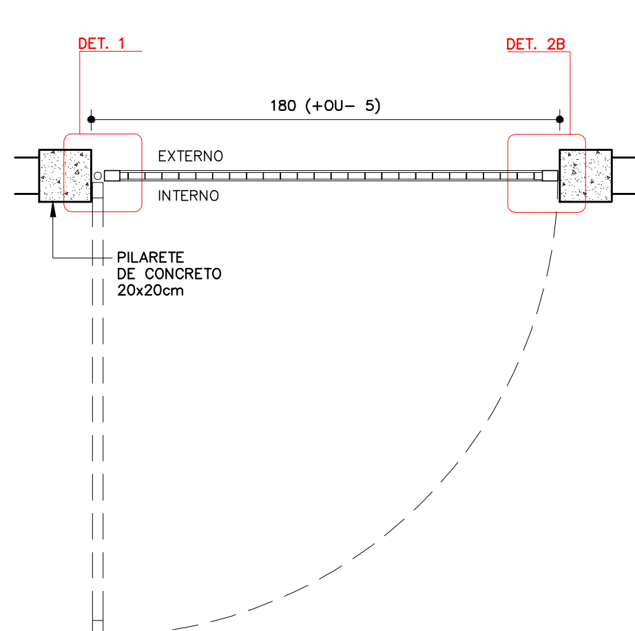
PLANTA PT-33
