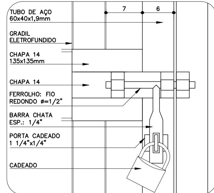
DETALHE 4A PT-35
