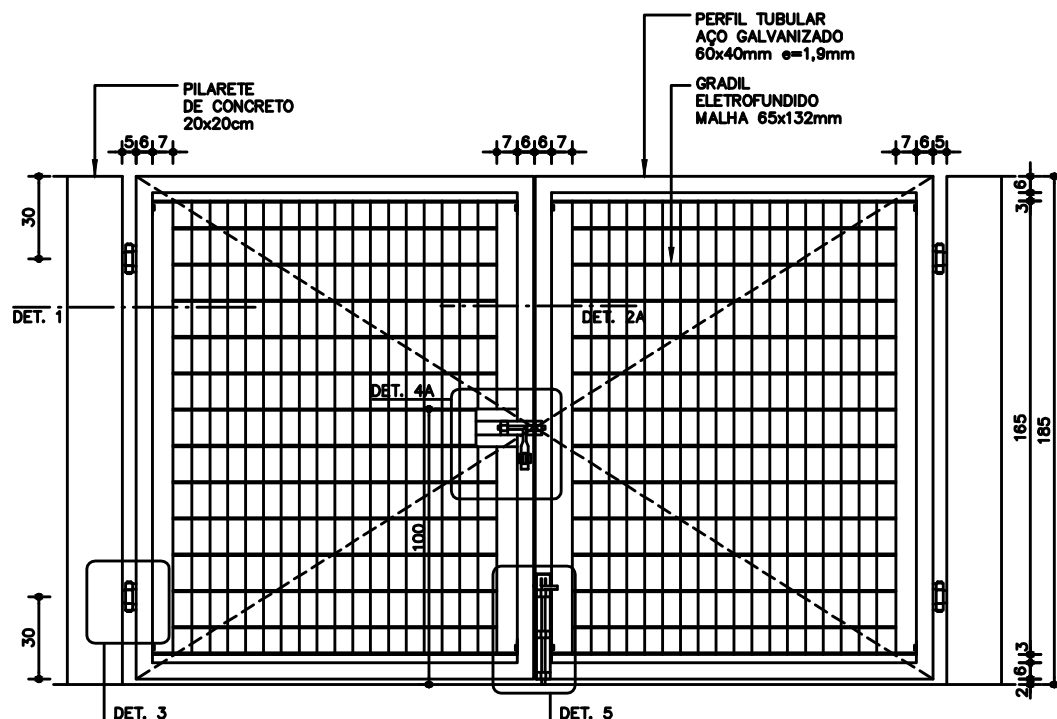
VISTA INTERNA PT-30
