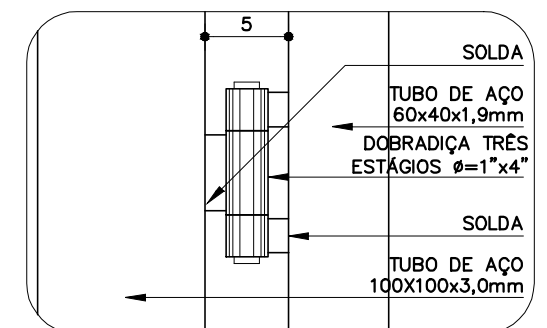
DETALHE 3 PT-35
