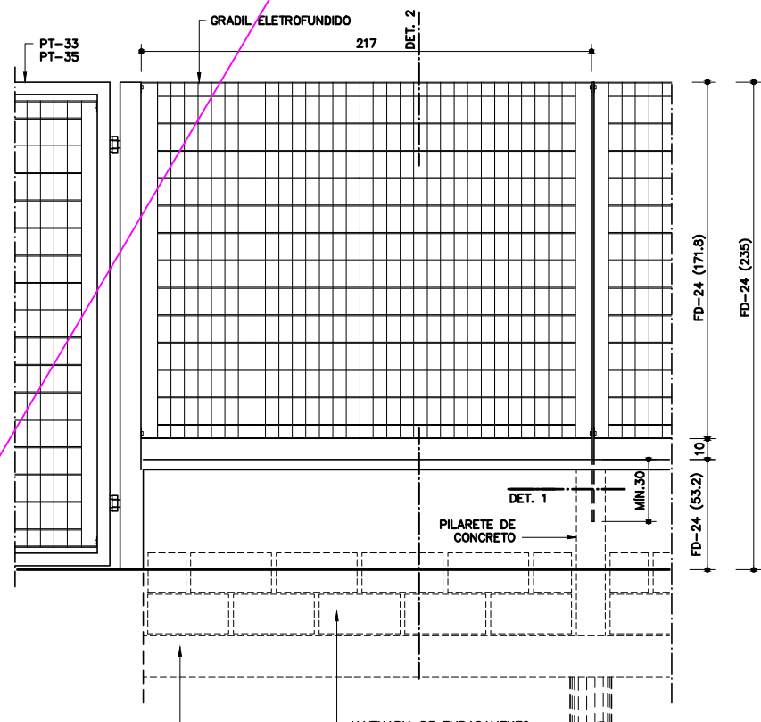
VISTA EXTERNA FD-24
