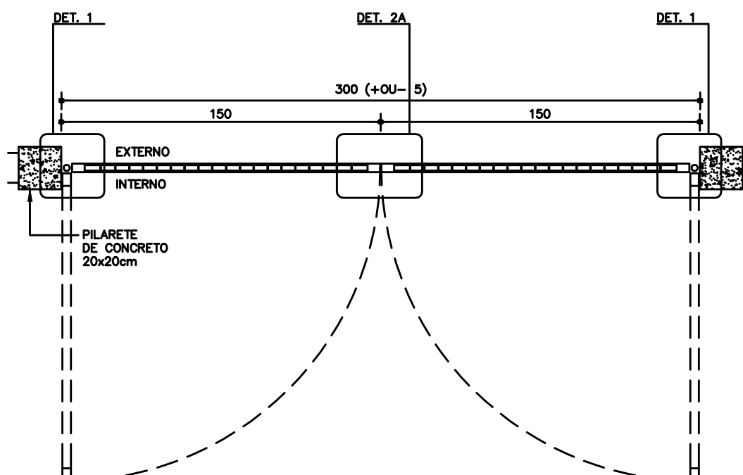
PLANTA PT-30
