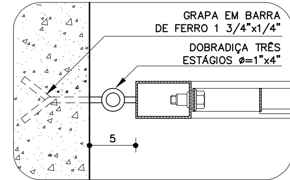
DETALHE 1 PT-33
