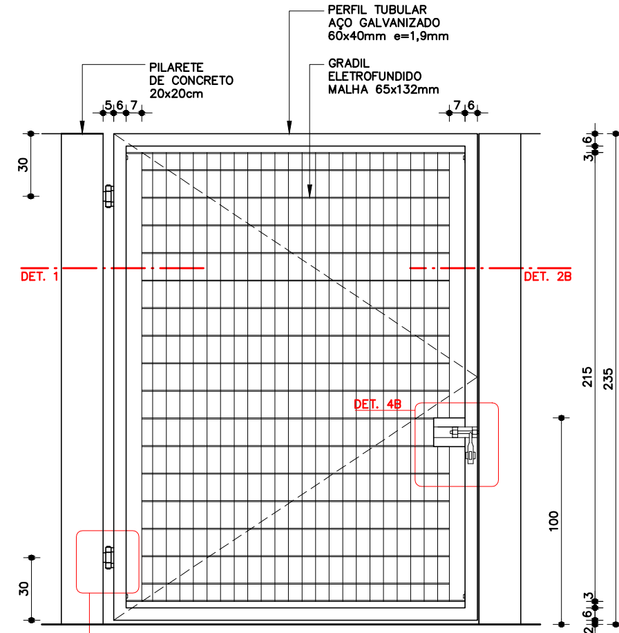
VISTA INTERNA PT-33
