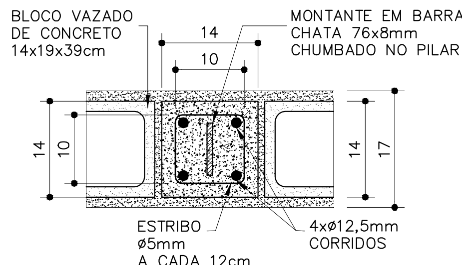
DETALHE 1 ESC. 1:10 FD-24
